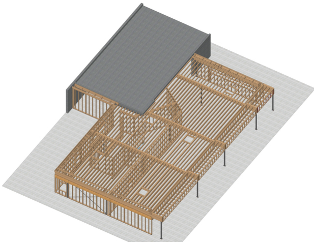
Konstruktionsansicht 3D
